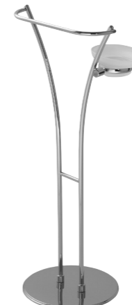
824 Piantana bidet Bidet stand Base Ø 210 L. 250 H. 610 mm
